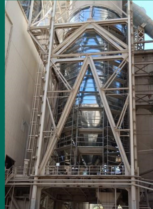
Rashladni toranj - poslije radova
